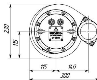
Гном 25-20Ех
