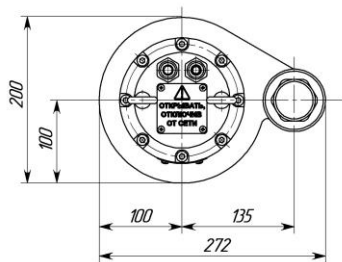
Гном 10-10Ех
